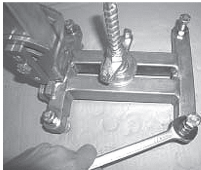
Юстировочные винты (контрагайки) на подножке P-3000-Profi Рис. 3.26
