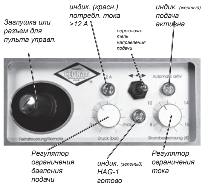
Органы управл. на доп. маслостанции HAG-1
