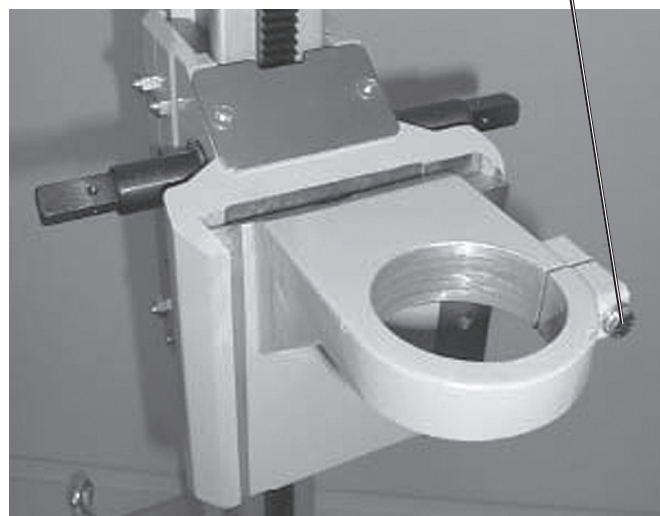
Пластина для моторов с шейкой крепления (тип В, 4831) смонтирована на салазки H-201 (позиция 1, аналог P-3000)
