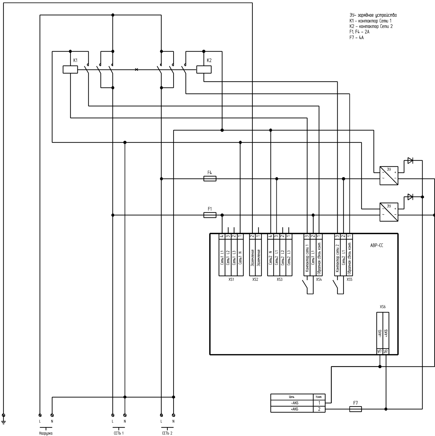
Рис. 6.4. Схема подключения АВР-СС для конфигурации АВР11 с общим нейтральным проводом
