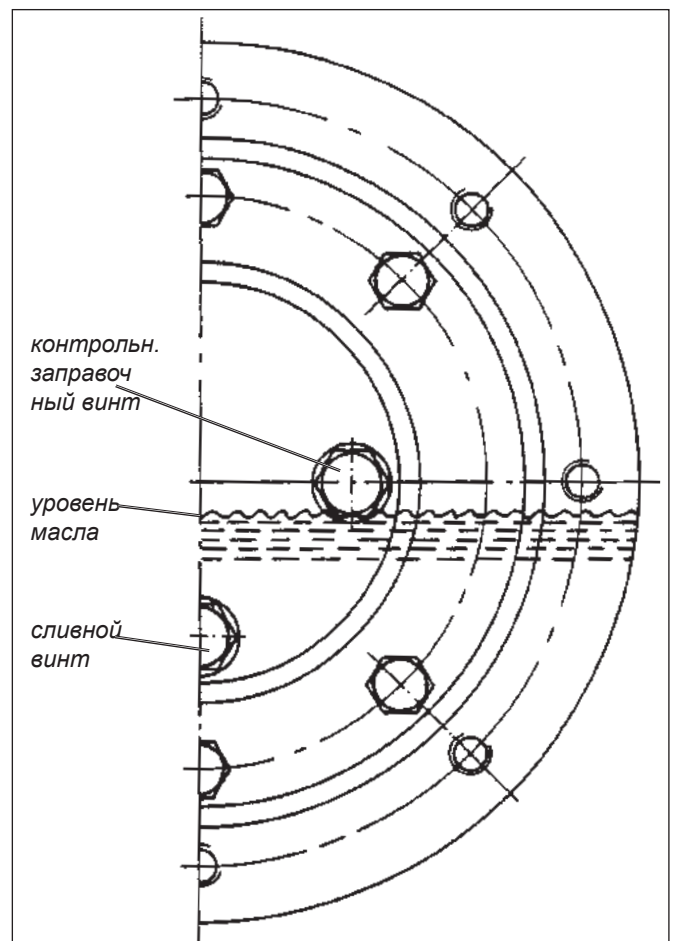
Положение редуктора ступиц колес CF - 6020 для контроля уровня масла и соотв. слива масла
