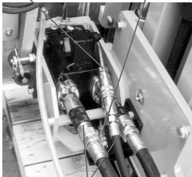
Двигатель привода диска, гидрошланги Рис. 7.4
