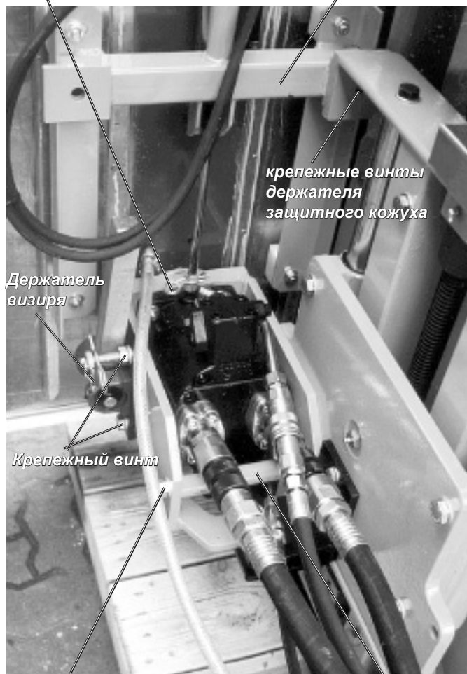
Режущая головка, двигатель привода диска слева Рис. 7.2
