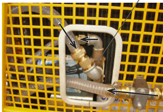
CF-6020 спереди, насос подключен для режима всасывания
