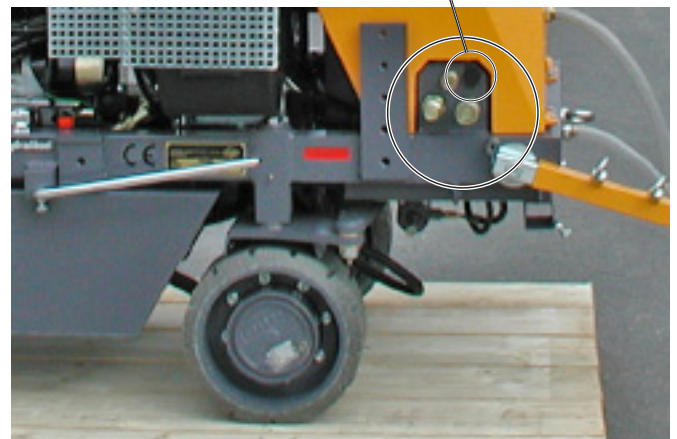
Разъемы доп. гидравлики (спереди, справа, прямой ход, обратный ход, утечное масло) Рис. 2.2
