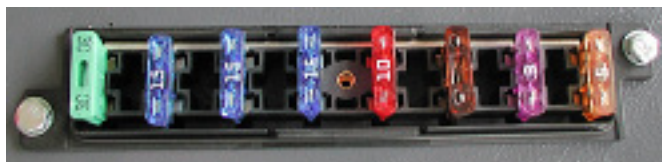
CF-6020 Блок предохранителей (крышка снята) Рис. 8.17
