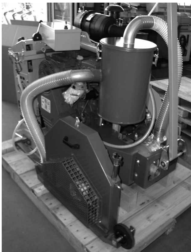
CF-3002 D, с доп.(со стороны инструмента) откач. приспособлением 4.3 и откач. кожухом Рис. 4.36
