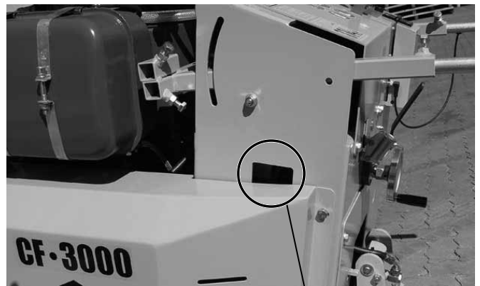
Корпус слева, отверстие для глазка уровня гидр. масла Рис. 4.8
