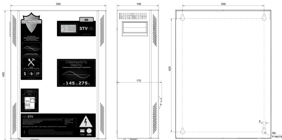
Рисунок 2 - Габаритные и установочные размеры STV-06, STV-08
