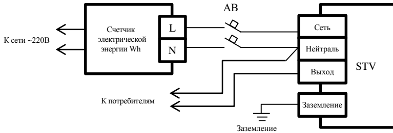
Рисунок 5 – Схема подключения
