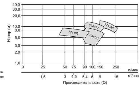
Диаграмма спектр моделей односкоростных насосов
