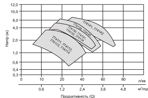
Діаграма спектр моделей трьохшвидкісних насосів
