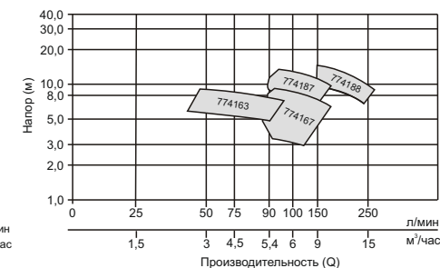
Диаграмма спектр моделей односкоростных насосов
