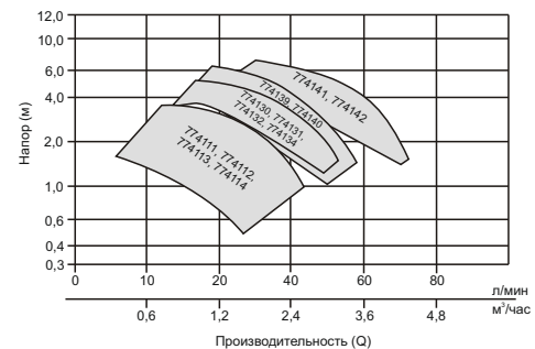
Диаграмма спектр моделей трехскоростных насосов
