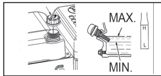
Motoröl-Einfüllschraube
