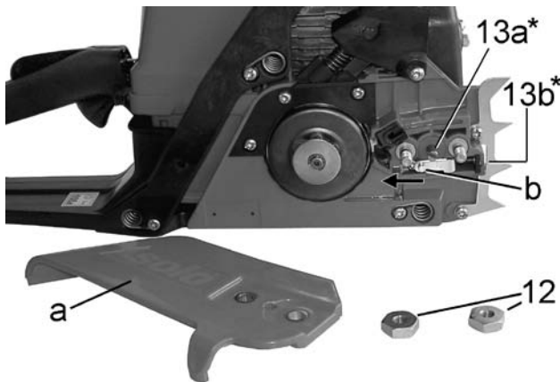
Рис. 2 (643 IP). 13a* - 636, 642, 643 IP 13b* - 635
