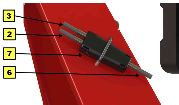
Obr. 12: Uchytení nože
