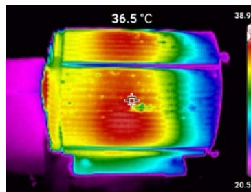
Инфракрасная термограмма электродвигателя, сделанная тепловизором Fluke TiS55+
