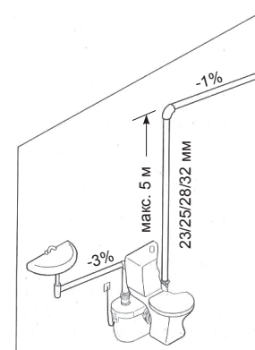
Рис. 2. Монтажная схема.
