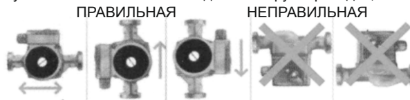
Рис. 3. Установка насоса.
