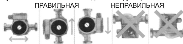
Рис. 3. Установка насоса.
