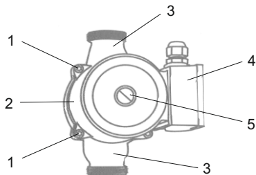
Рис. 1. Конструкция насоса.
