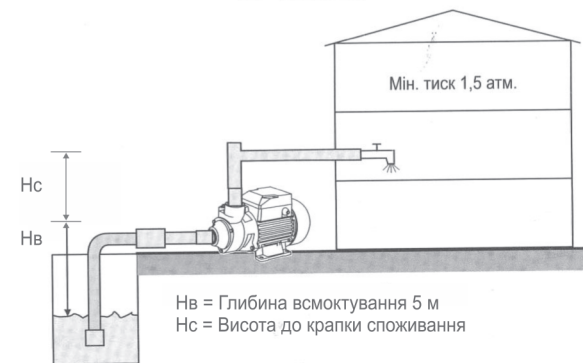
Мал. 1. Типові схеми водопостачання з використанням відцентрового поверхневого насоса.
