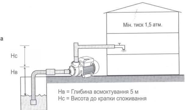
Мал. 1. Типові схеми водопостачання з використанням відцентрового поверхневого насосу.
