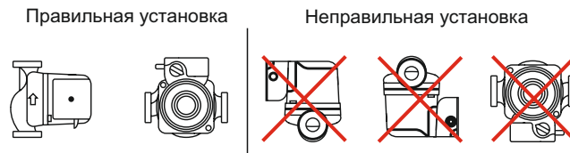
Рис. 3. Установка насоса.
