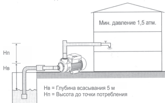
Рис. 1. Типовые схемы водоснабжения с использованием вихревого насоса.
