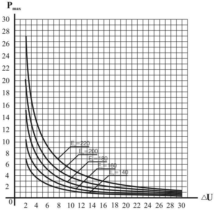
Рисунок 9. График зависимости максимальной мощности от падения напряжения в линии при испытательной нагрузке 1кВт. ДЛЯ ЗАМЕТОК
