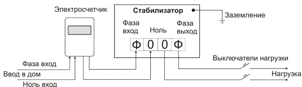
Рис.6 – Схема подключения стабилизатора к однофазной сети
