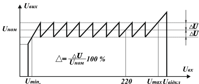
Малюнок 1. Загальна діаграма роботи нормалізатора.
